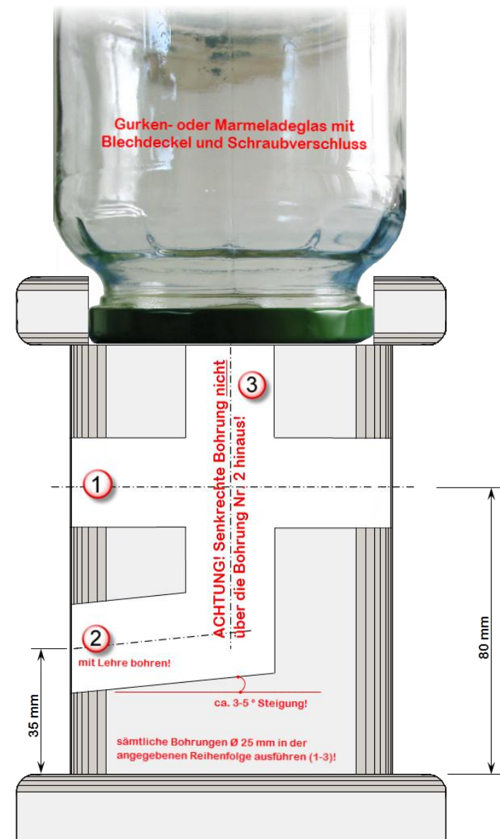
Seiten-Schnitt 1:1,5 (Bohrungen)
